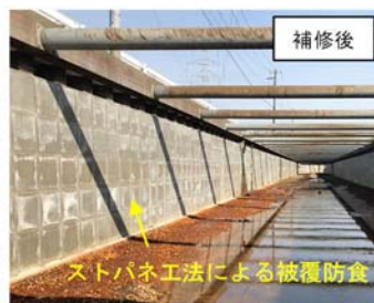
（ストパネ工法による補修）
